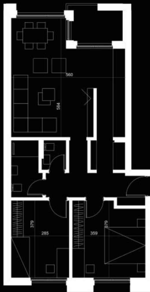
DIMENSIONET E NJËSISË B1
