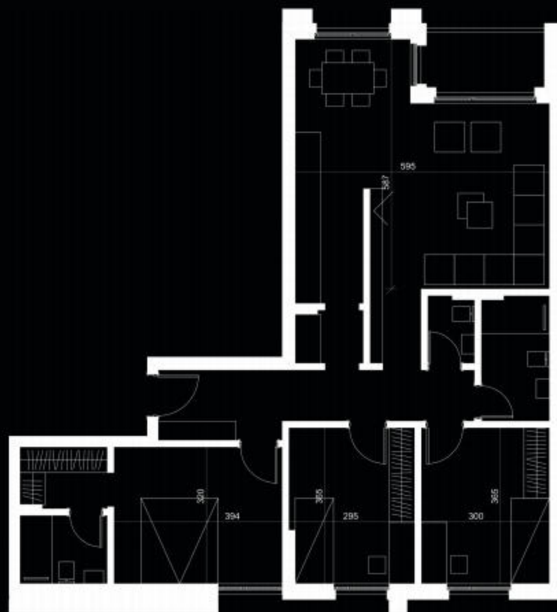
DIMENSIONET E NJËSISË A4
