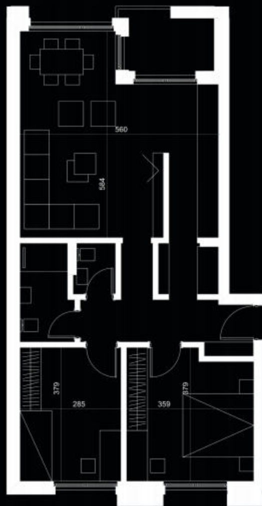
DIMENSIONET E NJËSISË A1
